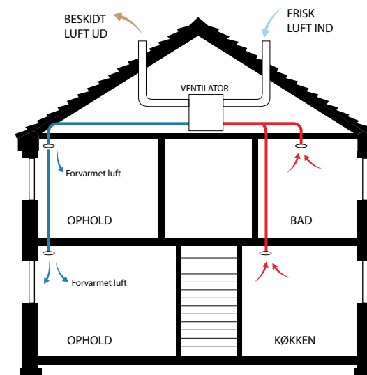
Princip for fremtidig ventilation som giver den nødvendige friskluftstilførsel og samtidig suger den beskidte luft ud fra køkken og bad.
